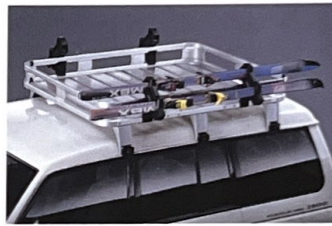
⑱ スキーアタッチメント ¥32,400(含む参考取付工賃¥2,400)MZ535886 ●ヘビーデューティーキャリアのサイドに固定するタイプ。樹脂製。キーロック付。スキー4セットが積めます。
